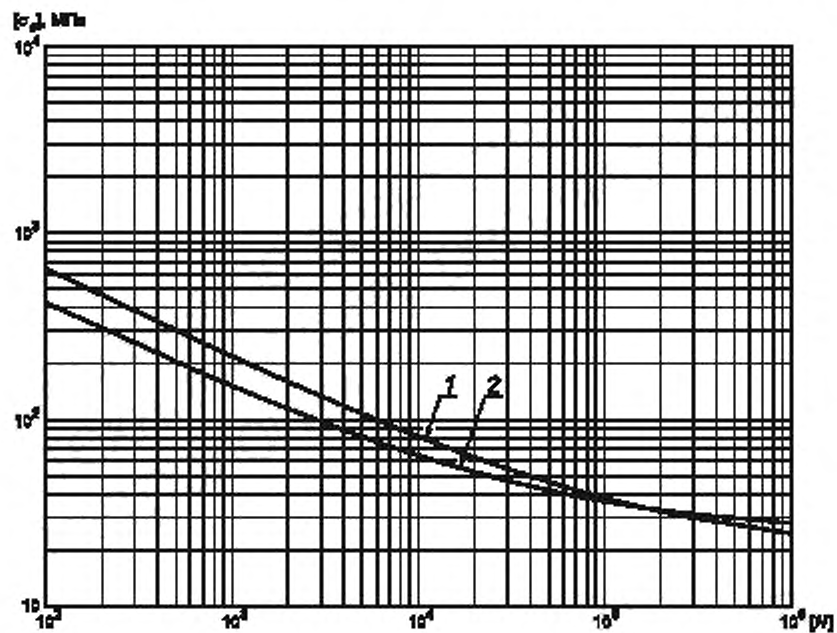
Рисунок 8 — Расчетная кривая усталости для сплавов титана
