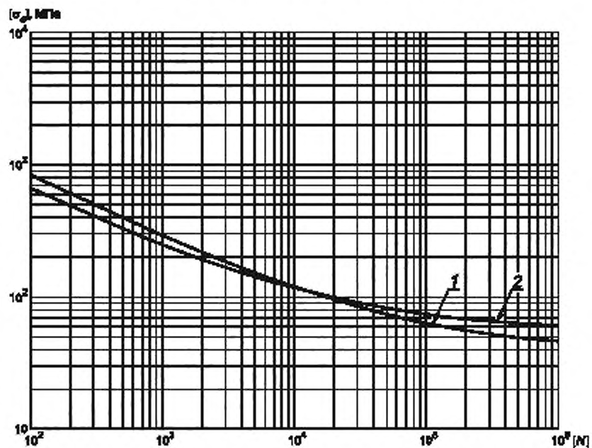
Рисунок 6 — Расчетная кривая усталости для сплавов алюминия
