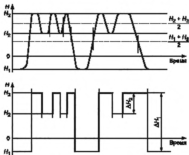
Рисунок 1. лист 1 — Эпюры циклов нагружения
